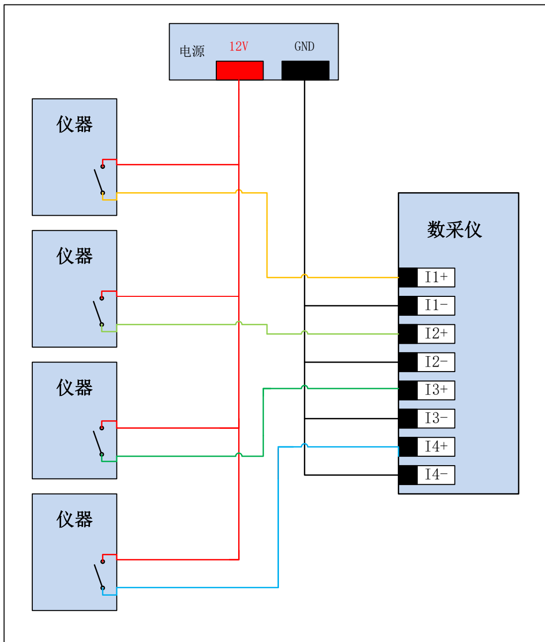
开关量输入接线示意图
